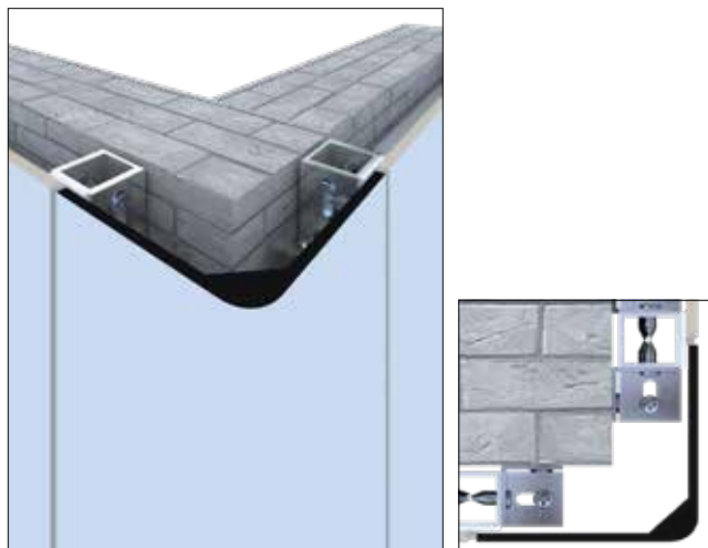
1. 倍耐板阳角
