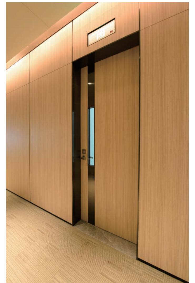
墙面板 U 型装饰条，转角为金属海棠角
