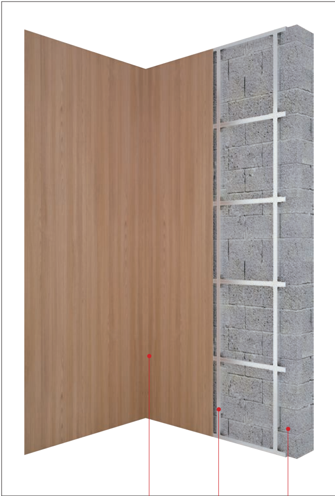
保特耐饰材 铝合金龙骨 砌体基墙
